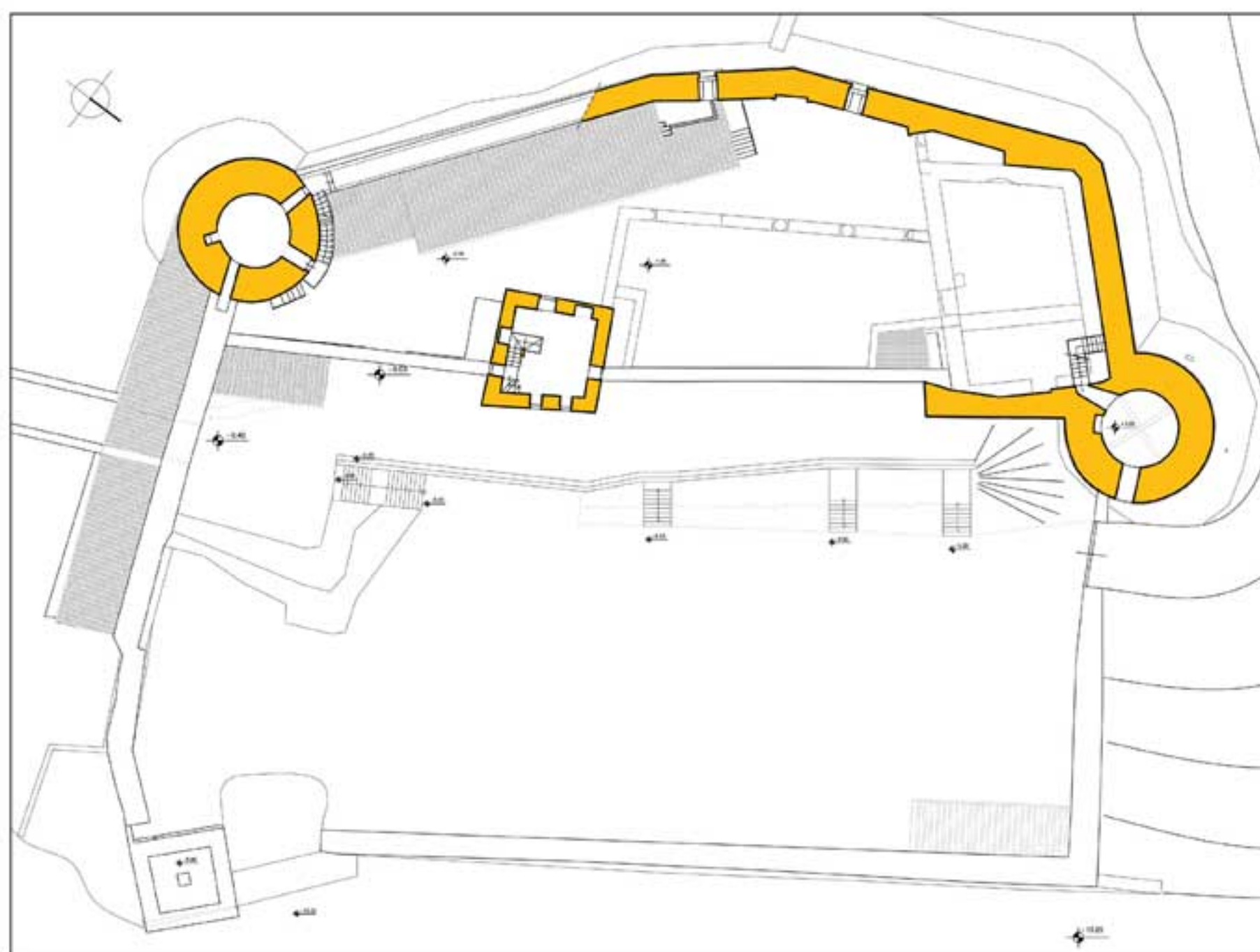
pianta piano quota +5,00 m
